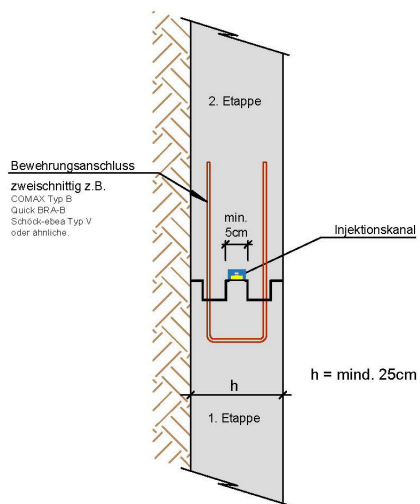
Arbeitsfuge mit Bewehrungsanschluss
